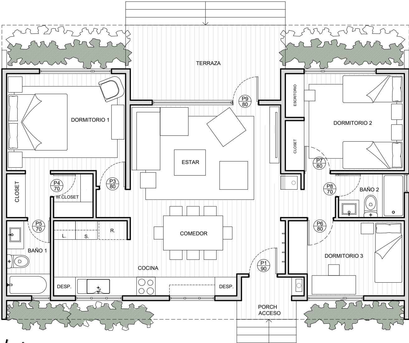
PLANTA ARQUITECTURA
