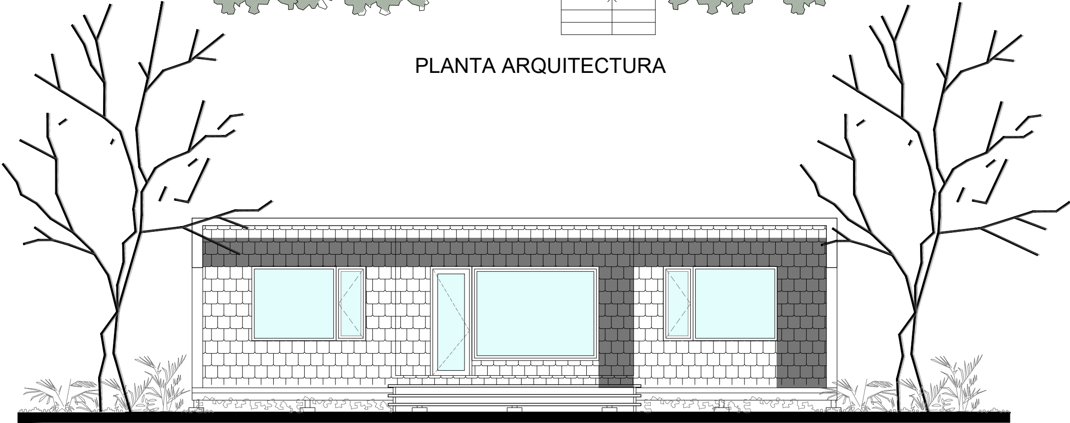
ELEVACION JARDIN
